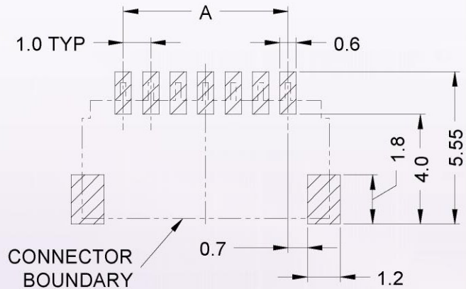
P.C.B PATTERN DIMENSION
